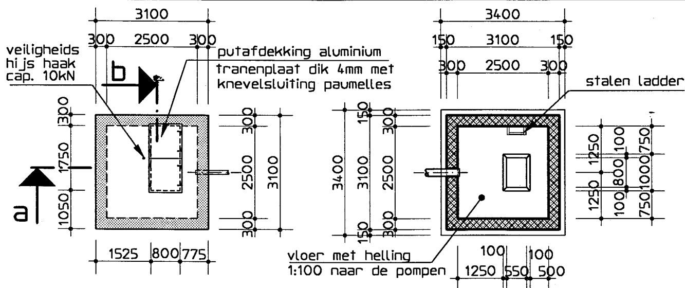
Bovenaanzicht put 1:100
