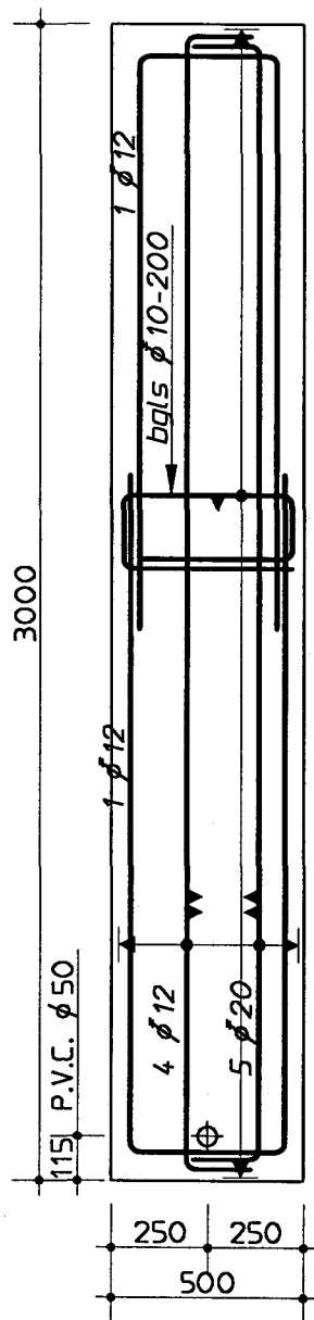
Dwarsdoorsnede
