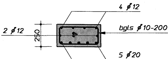
Dwarsdoorsnede
